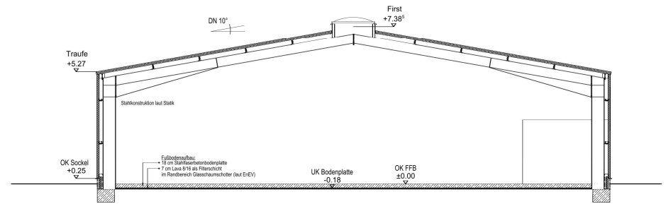
Schnitt A-A
