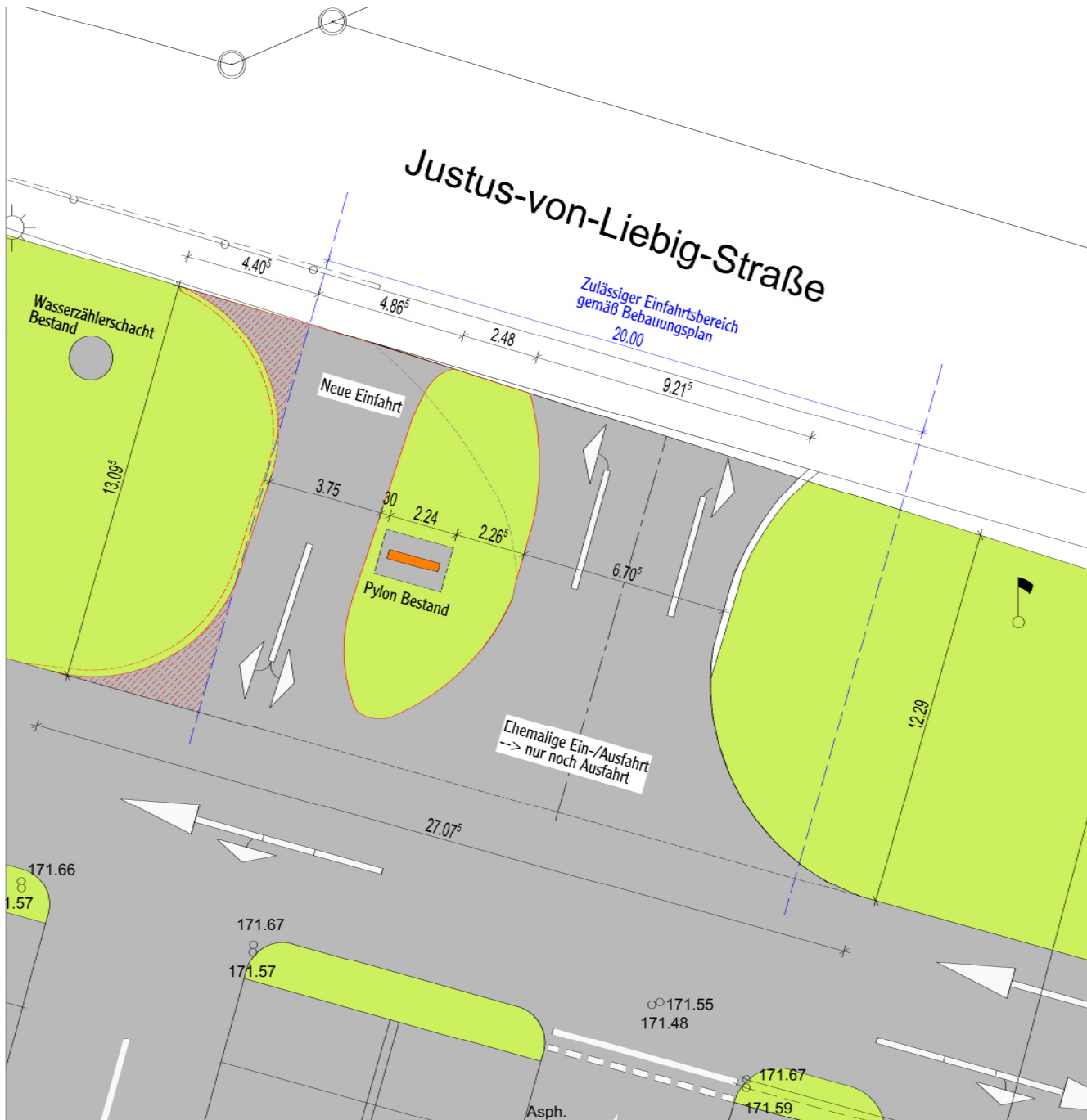
Ausschnitt Freiflächenplan - Einfahrt Grundstück Neuplanung Erweiterung
