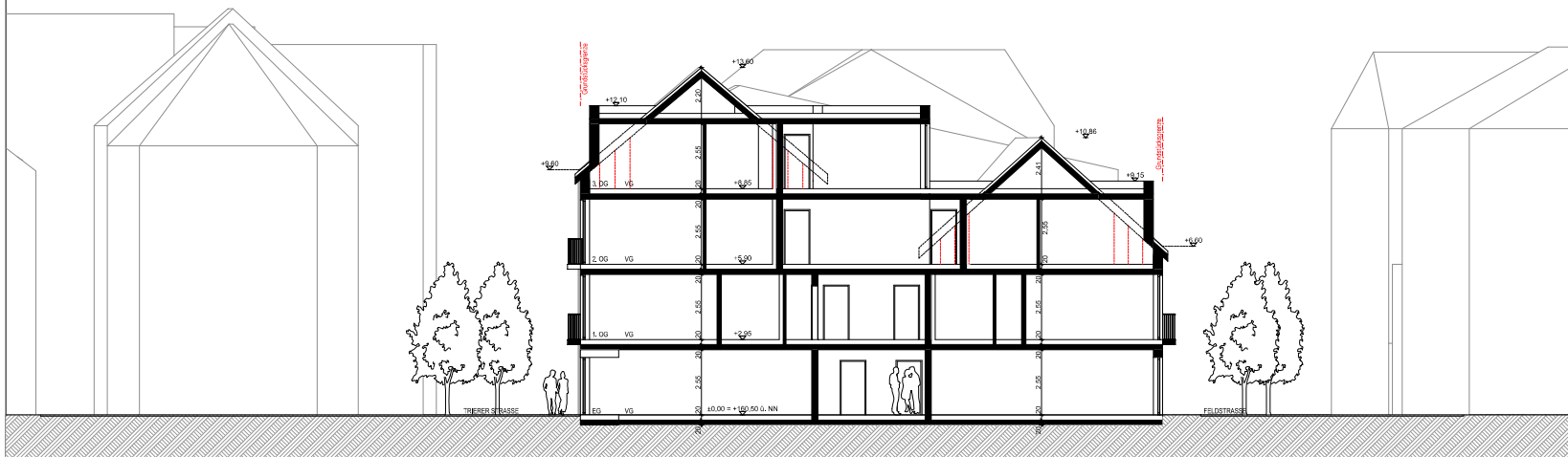
SCHNITT A-A 1.100
