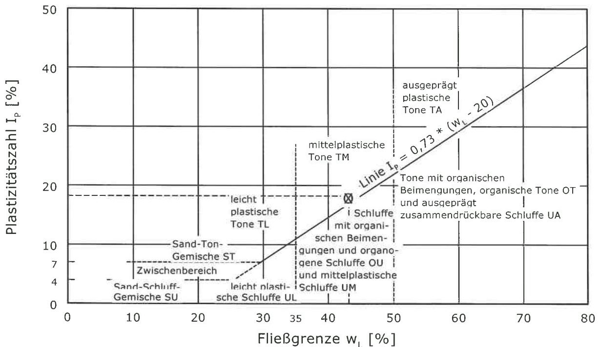
Plastizitätsdiagramm
