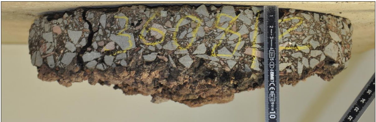
Foto 4: Erkundungsstelle 2 – Bohrkernprobe
