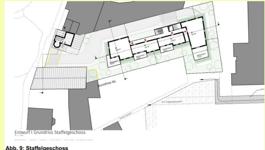
Abb. 9: Staffelgeschoss
