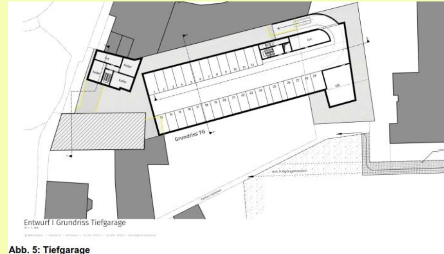
Abb. 5: Tiefgarage
