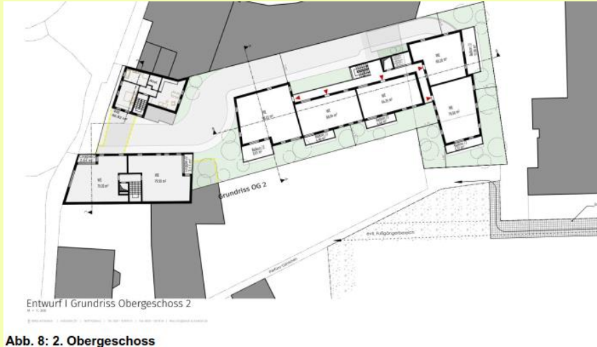
Abb. 8: 2. Obergeschoss
